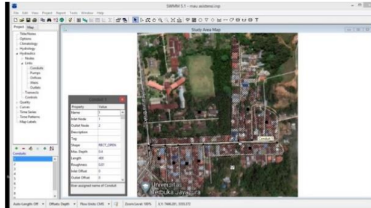
Fig 6: Display image conduit
