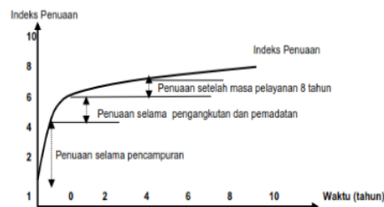
Gambar 1. Kecepatan penuaan aspal ( Shell Bitumen Handbook , 2015 [21])
