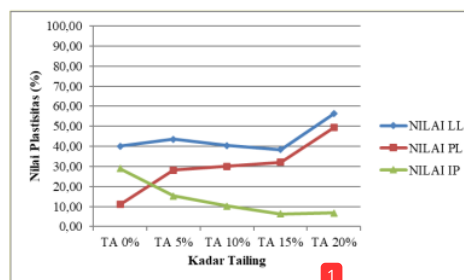
Gambar 3. Grafik Hubungan antara nilai batas cair, batas plastis dan indeks plastisitas
