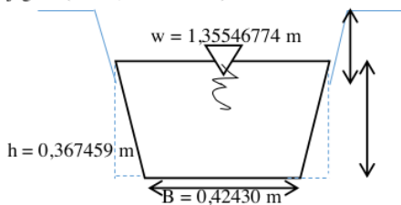
Gambar 3. Dimensi Saluran Drainase KrI yang direkomendasikan (hitungan)
