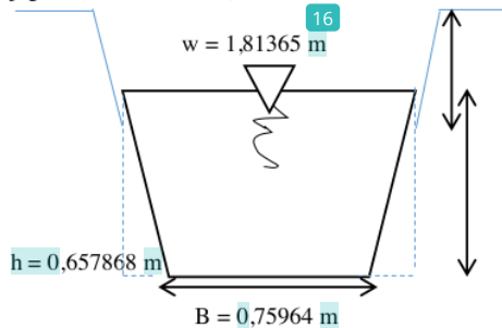
Gambar 4. Dimensi Saluran Drainase KrII yang direkomendasikan (hitungan)
