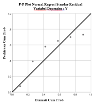
Gambar 4.1. Grafik model uji normalitas
